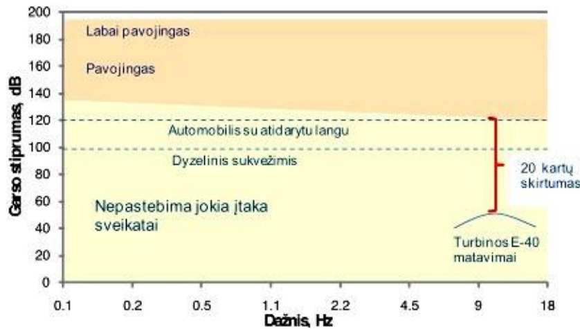
3 pav. Vėjo elektrinių ir kitų šaltinių sukeliamas infragaras. Šaltinis: www.wind-energie.de
